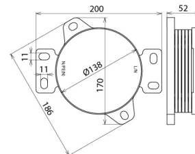
Maßbild DSO 1 255
