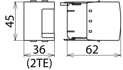
Maßbild DSE MOD 242
