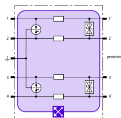
Principalschaltbild BXT ML4 BD HF 24
