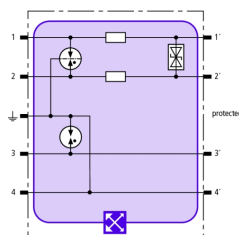
Principalschaltbild BXT ML2 BD HFS 5
