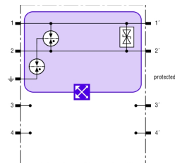
Principalschaltbild BXT ML2 BD HF EX 6
