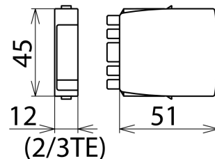
Maßbild BXT ML2 BD HF EX 6
