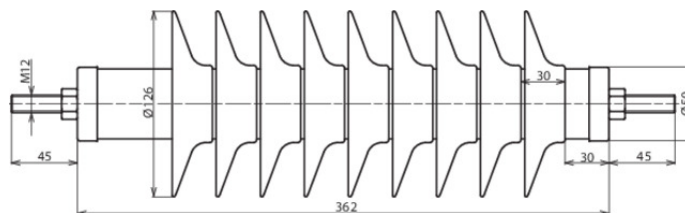
Maßbild DMI 36 10 1 H
