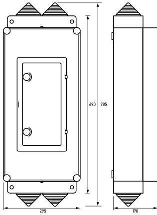
Maßzeichnung Gruppenansicht
