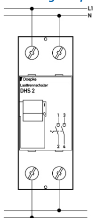
Anschlussschema
