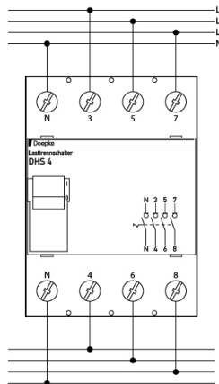
Anschlussschema
