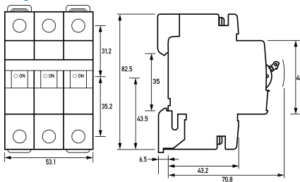
Maßzeichnung Gruppenansicht
