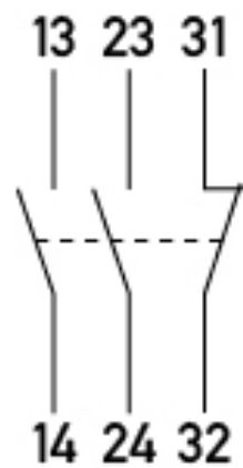
Anschlussschema
