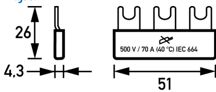
Maßzeichnung Gruppenansicht
