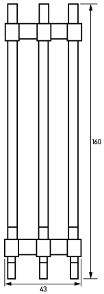
Maßzeichnung Gruppenansicht
