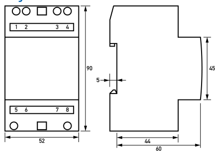
Maßzeichnung Gruppenansicht
