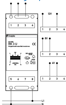
Anschlusschema
