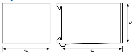
Maßzeichnung Gruppenansicht
