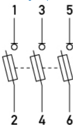
Anschlussschema
