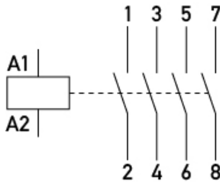
Anschlussschema
