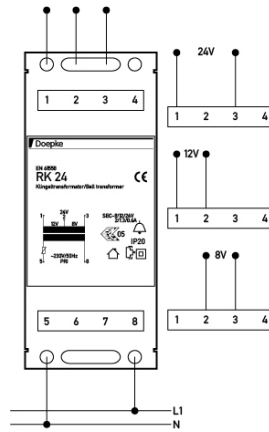
Anschlussschema
