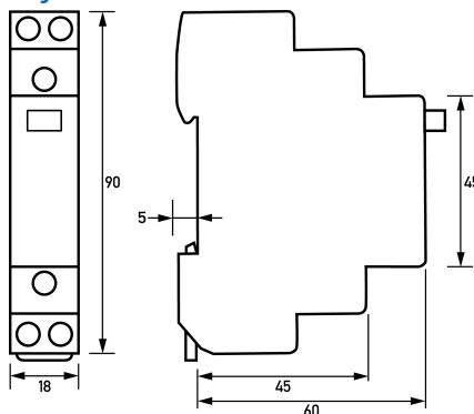
Maßzeichnung Gruppenansicht
