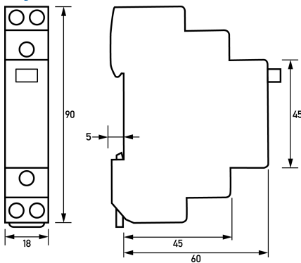
Maßzeichnung Gruppenansicht
