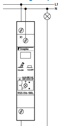
Anschlussschema
