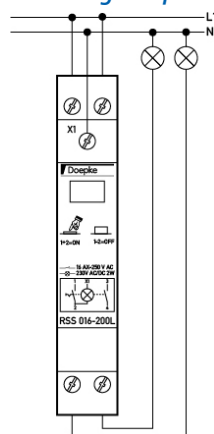
Anschlussschema
