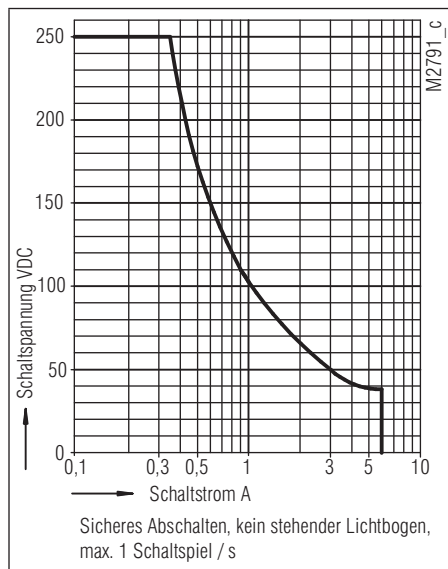
Lichtbogengrenzkurve
