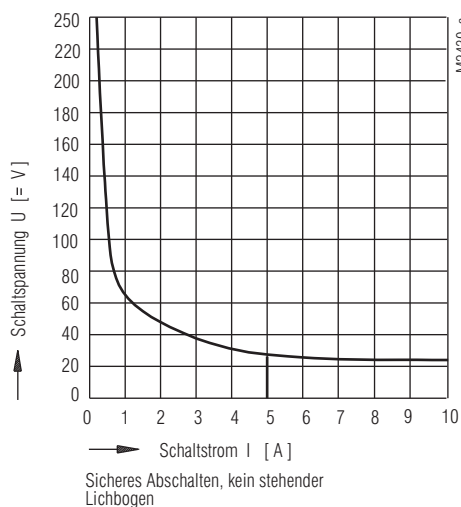
Lichtbogengrenzcurve
