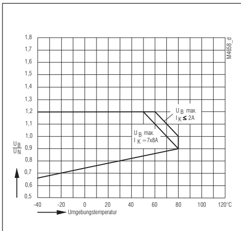
Betriebsspannungs-Grenzcurve ohne Einfluss durch Eigenerwärmung umgebener Bauteile
