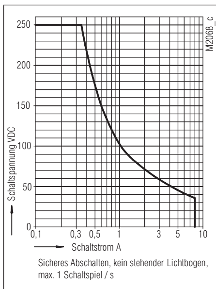
Lichtbogengrenzkurve (Lastgrenzkurve)
