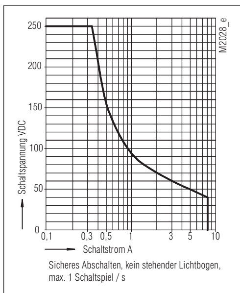
Lichtbogengrenzkurve (Lastgrenzkurve)
