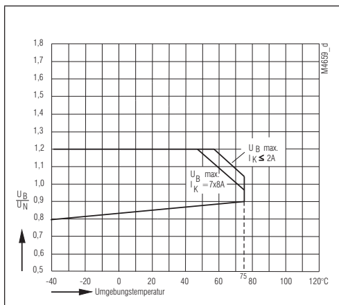
Betriebsspannungs-Grenzkurve ohne Einfluss durch Eigenerwärmung umgebener Bauteile
