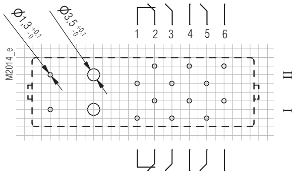
Anschlussbelegung OA5602.54 4S/2Ö
