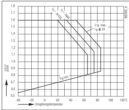
Betriebsspannungs-Grenzkurve OA 5601
