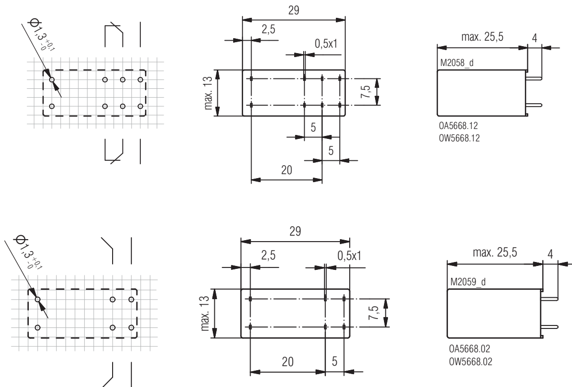
Bohrbild (Lötseite)
