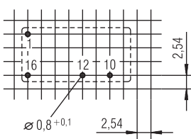
Bohrbild (Lötseite)
