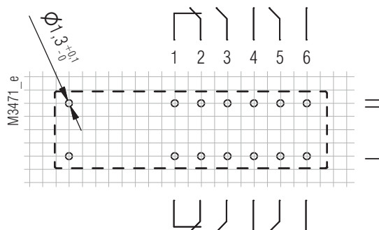
Anschlussbelegung OA 5612.50/...L4 2S / 4Ö
