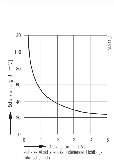
Lichtbogengrenzkurve (bei t_u = 20^\circ\text{C} ) für OW 5691 und OW 5699
