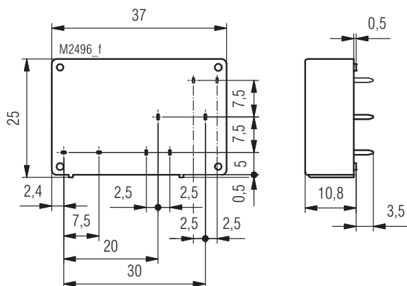
Bohrbild (Lötseite)
