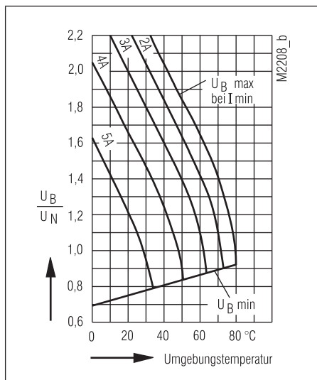
Betriebsspannungs-Grenzcurve
