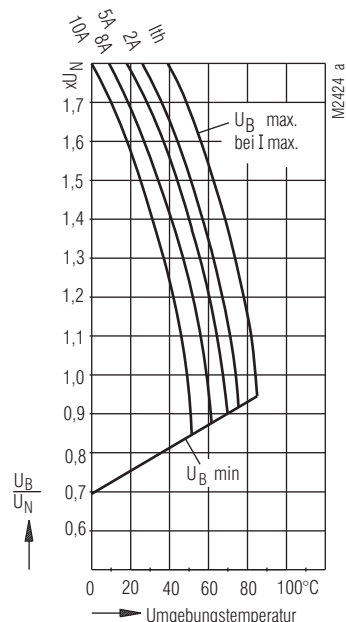
Betriebsspannungs-Grenzcurve OA 5690.11 10 A - Version
