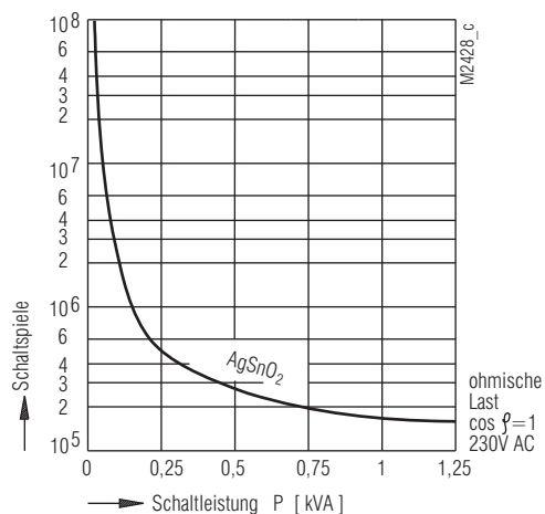
Kontaktlebensdauer OA 5690.11 5 A - Version
