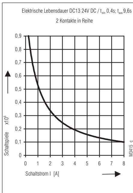
Elektrische Lebensdauer
