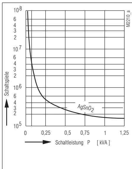
Kontaktlebensdauer
