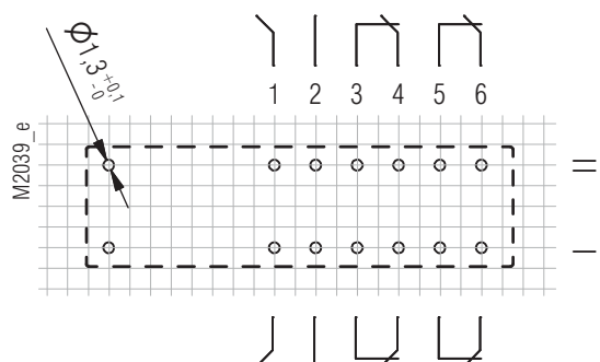
Anschlussbelegung OA 5612.50/...S1 2S / 4Ö
