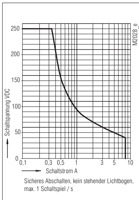
Lichtbogengrenzkurve
