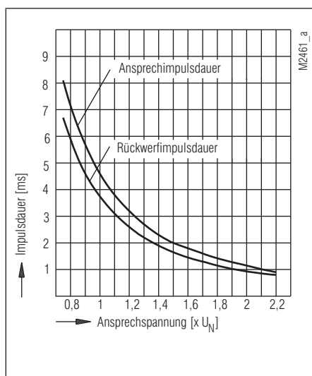
Ansprech-/Rückwerf-Impulsdauer
