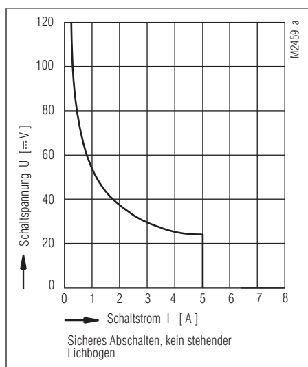
Lichtbogengrenzkurve (Lastgrenzkurve)
