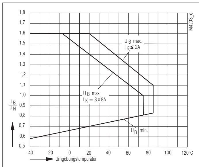
Betriebsspannungs-Grenzkurve OA 5642.48
