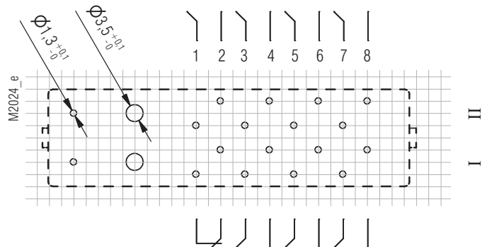
Anschlussbelegung OA5603.63 7S/1Ö
