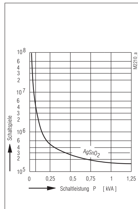
Kontaktlebensdauer (bei t u = 20°C)
