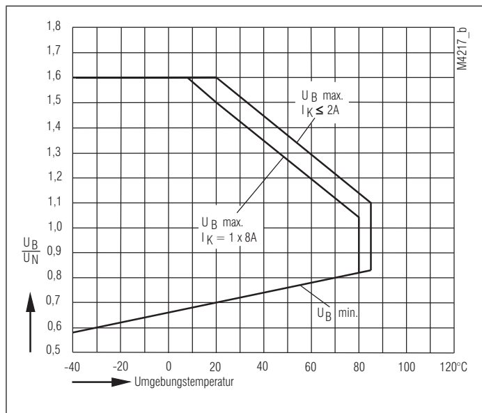
Betriebsspannungs-Grenzkurve OA 5642.16
