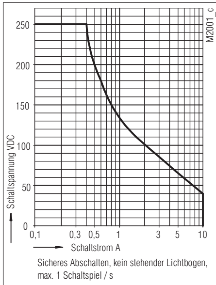
Lichtbogengrenzkurve
