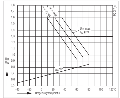
Betriebsspannungs-Grenzkurve OA 5603
