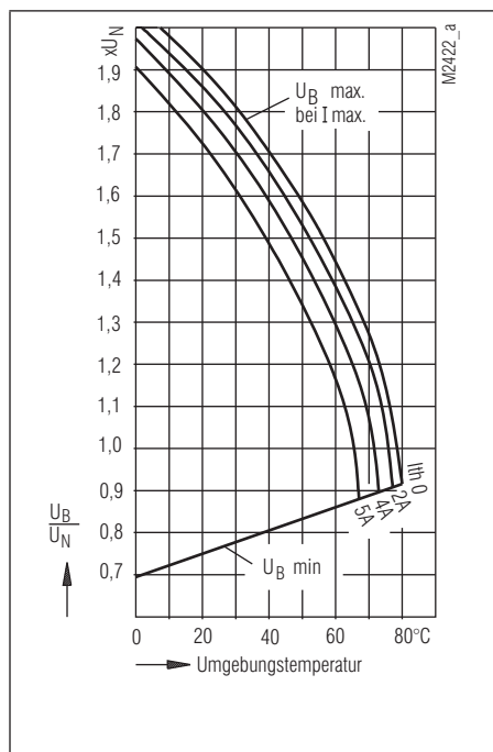
Betriebsspannungs-Grenzkurve
