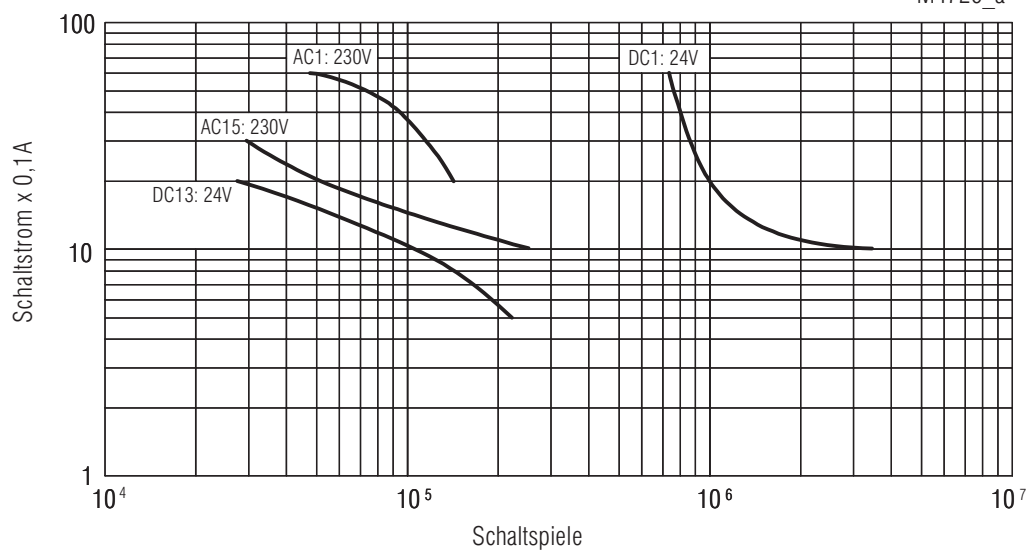
Elektrische Lebensdauer
