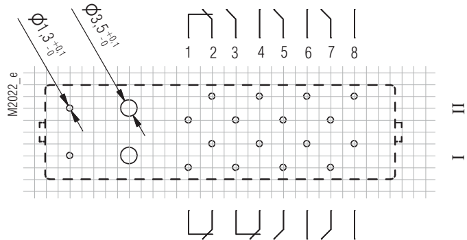
Anschlussbelegung OA5603.58 5S/3Ö
