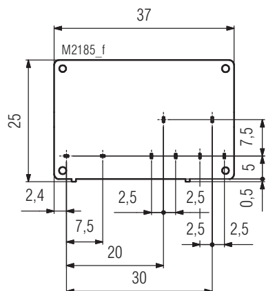
Bohrbild (Lötseite)
