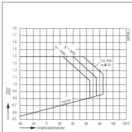
Betriebsspannungs-Grenzkurve OA 5612
