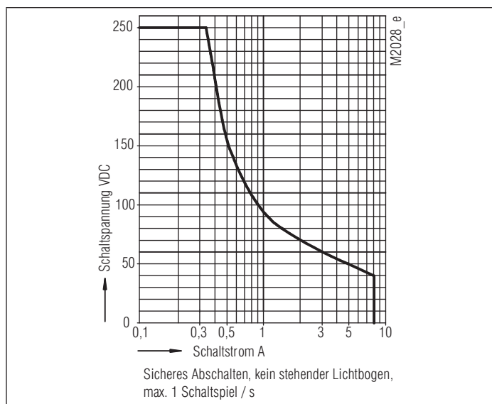
Lichtbogengrenzkurve (Lastgrenzkurve)
