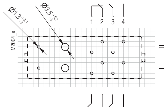
Anschlussbelegung OA5601.48 3S/1Ö
