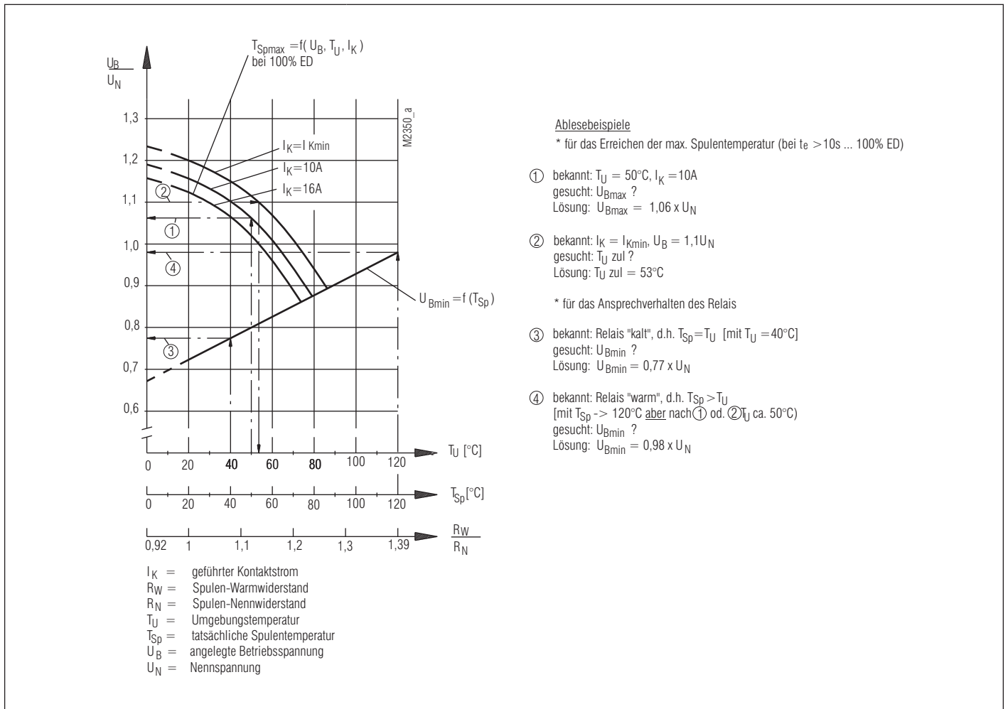
Betriebsspannungs-Grenzcurve
