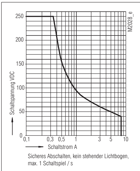
Lichtbogengrenzcurve (Lastgrenzkurve)
