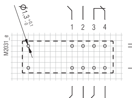
Anschlussbelegung OA 5611.28 1S / 3Ö
