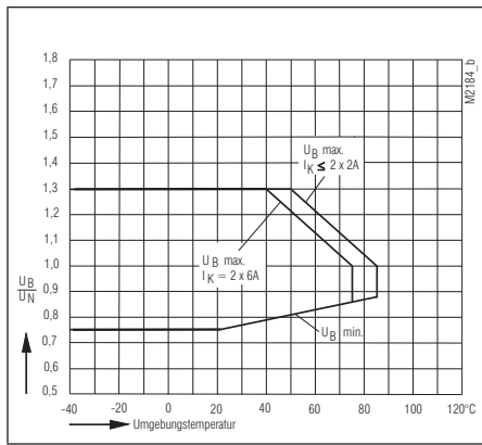
Betriebsspannungs-Grenzkurve
