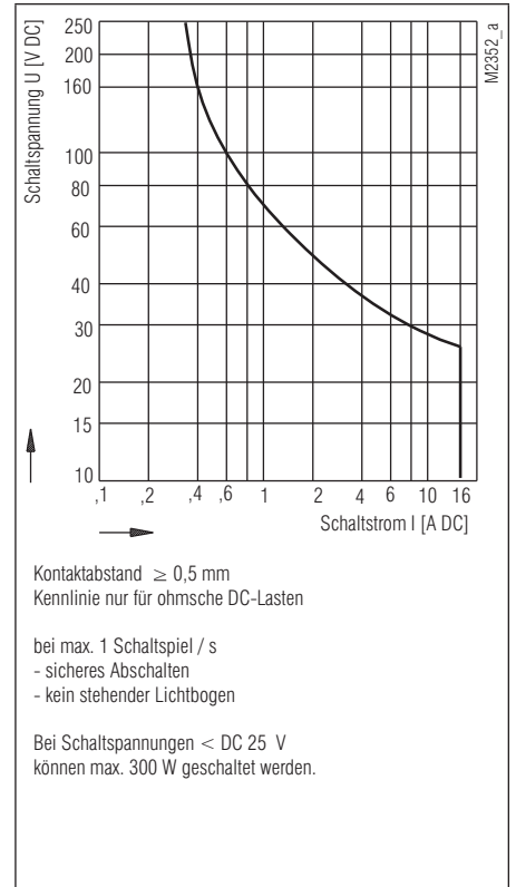
Lichtbogengrenzcurve
