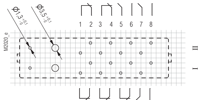
Anschlussbelegung OA5603.56 3S/5Ö
