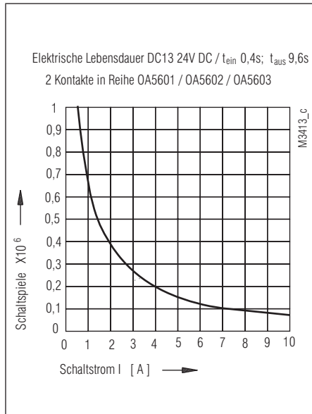
Elektrische Lebensdauer
