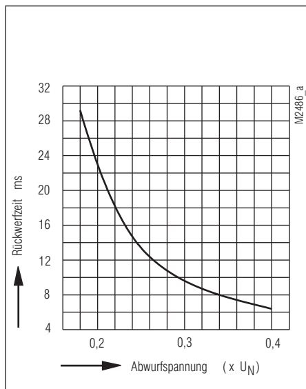
Rückwurfzeit
