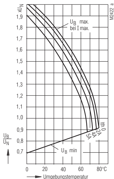
Betriebsspannungs-Grenzcurve OA 5690.11 5 A - Version
