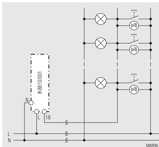
3-Leiter-Schaltung (L-getastet)
