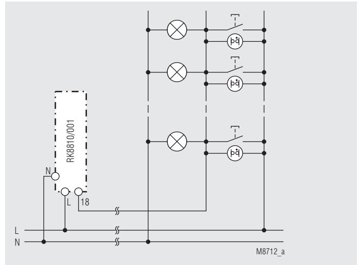
3-Leiter-Schaltung (L-getastet)
