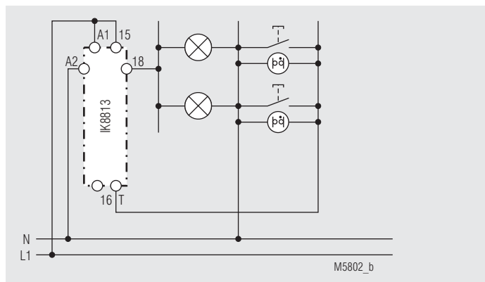
IK 8813 3-Drahtschaltung (ausschaltbar)
