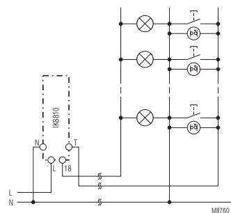
3-Leiter-Schaltung (N-getestet)
