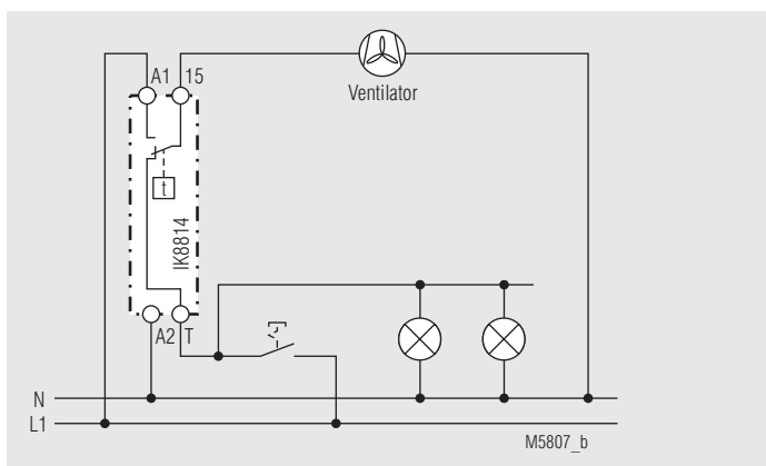
IK 8814 Nachlaufschaltung
