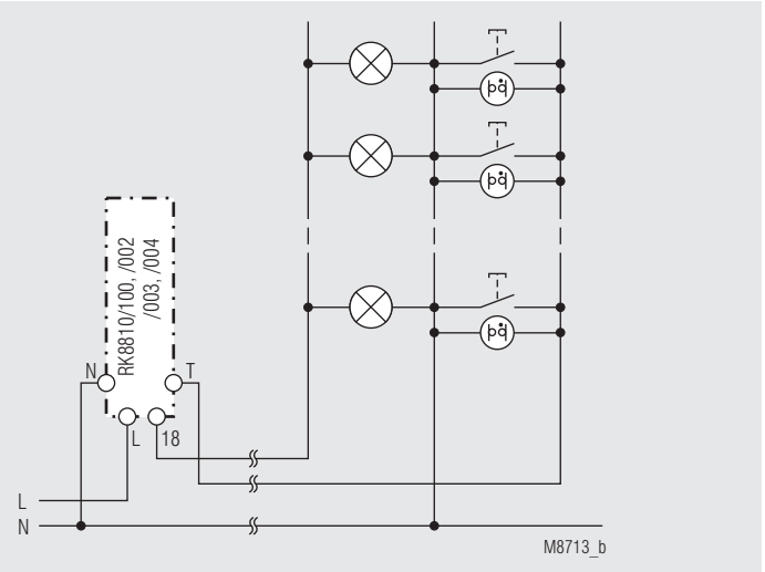
3-Leiter-Schaltung (N-getastet)
