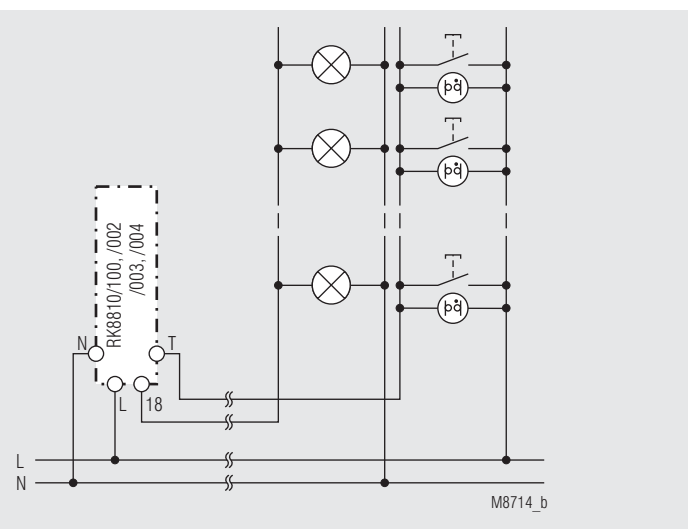
4-Leiter-Schaltung (L-getastet)
