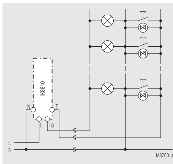
3-Leiter-Schaltung (N-getastet)
