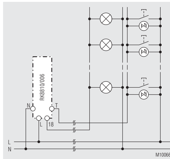
4-Leiter-Schaltung (L-getastet)
