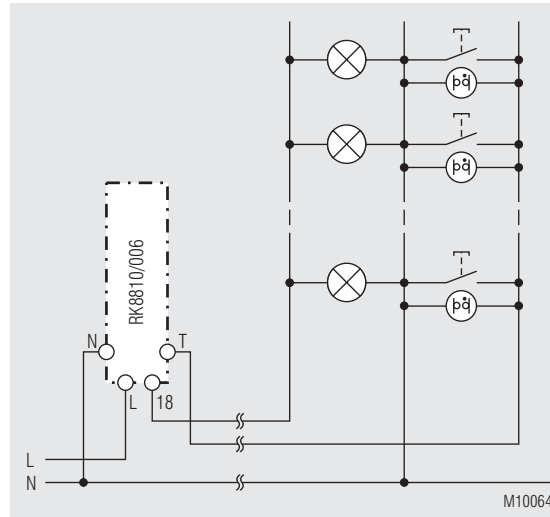
3-Leiter-Schaltung (N-getastet)
