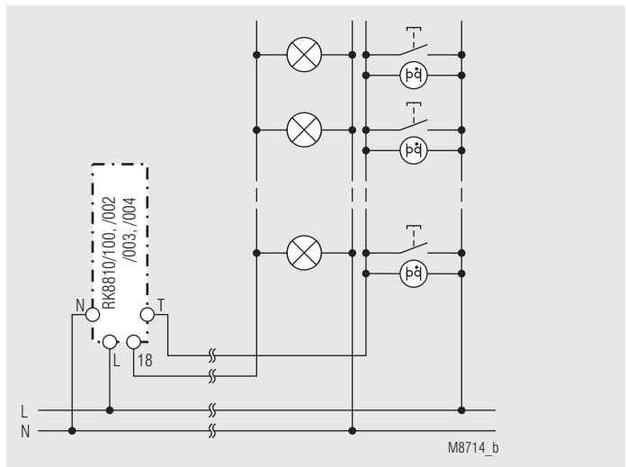
4-Leiter-Schaltung (L-getastet)
