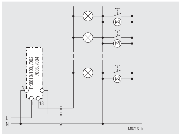
3-Leiter-Schaltung (N-getastet)
