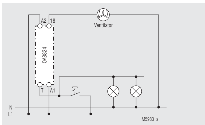
OA 8824 Nachlaufschaltung
