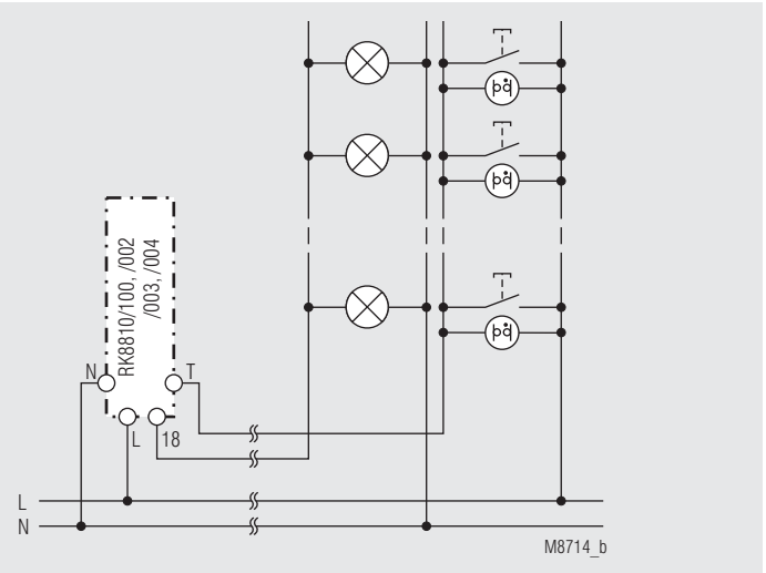
4-Leiter-Schaltung (L-getastet)
